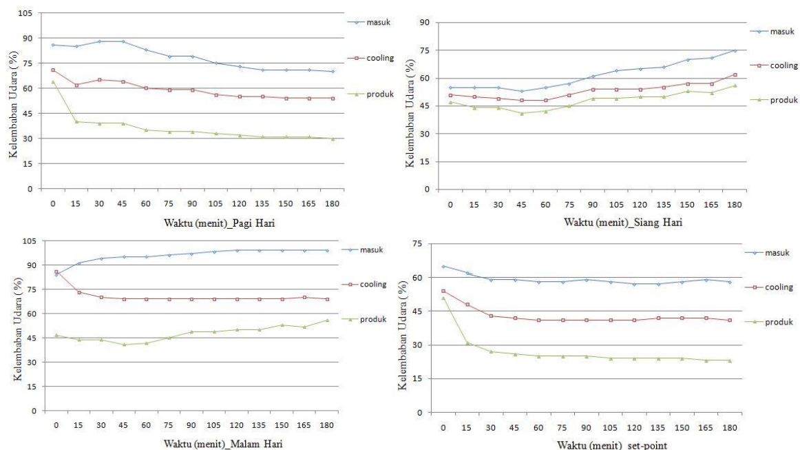
Gambar 5 Perbandingan nilai kelembaban relatif (%RH) udara terhadap waktu
