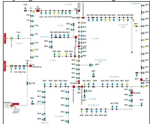
Gambar 2. Single line diagram jaringan distribusi 20 kV penyulang Jambi
