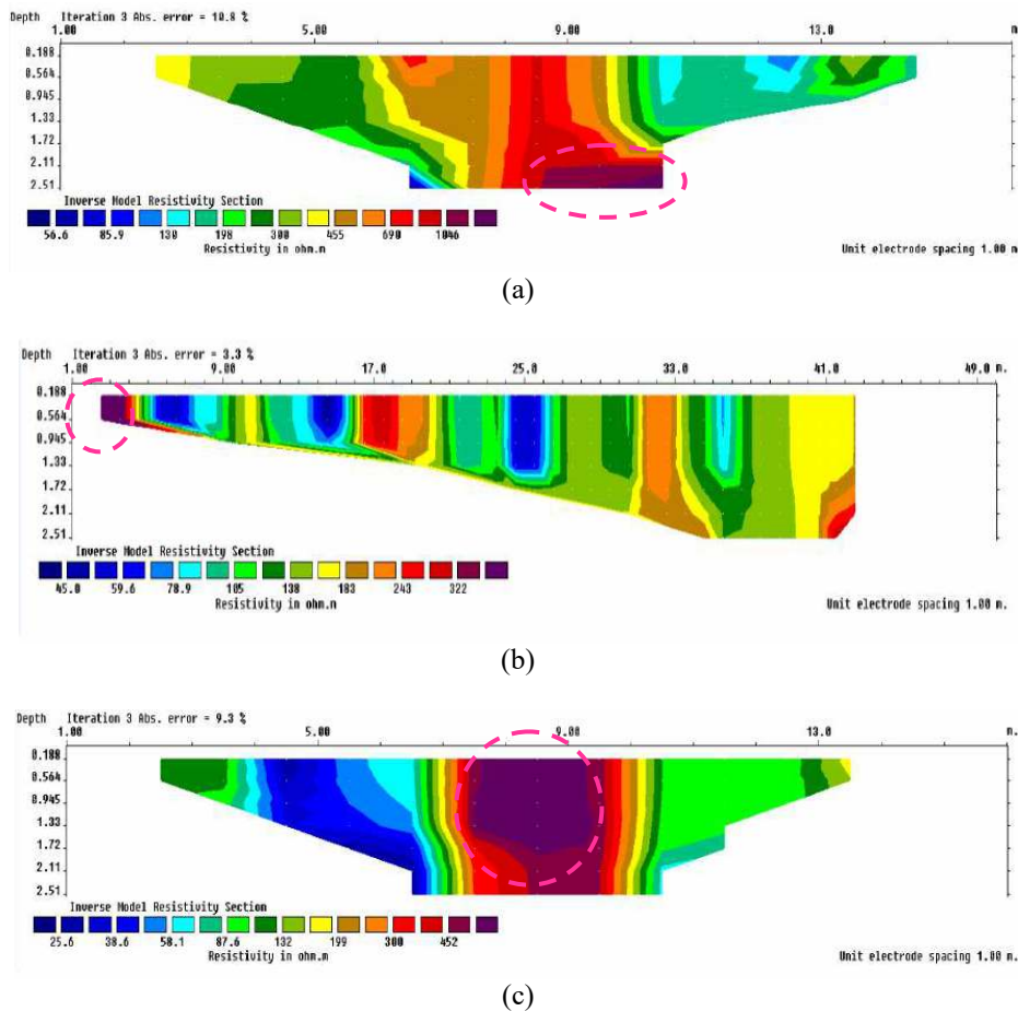
Gambar 2. Interpretasi data pengukuran menggunakan metode geolistrik resistivity : (a) Struktur bawah permukaan Lintasan 1 (Pitulima, 2016), (b) Struktur bawah permukaan Lintasan 2 (Pitulima, 2016), (c) Struktur bawah permukaan Lintasan 3 (Pitulima, 2016).
