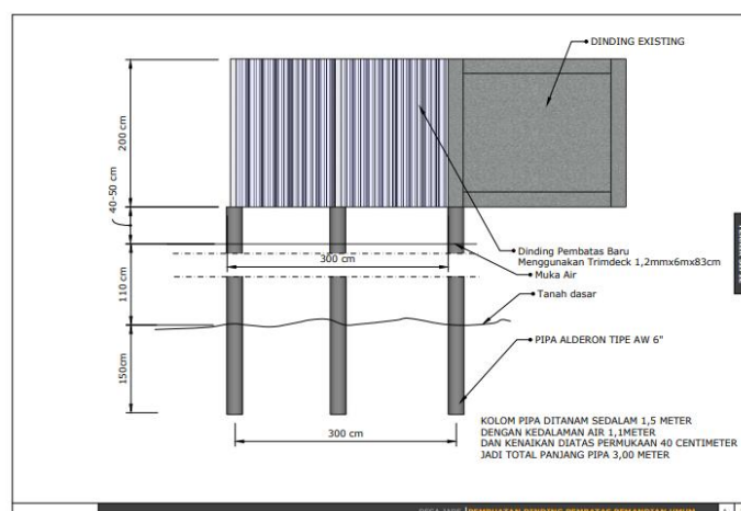
Gambar 3. Desain tiang pondasi tempat pemandian umum
