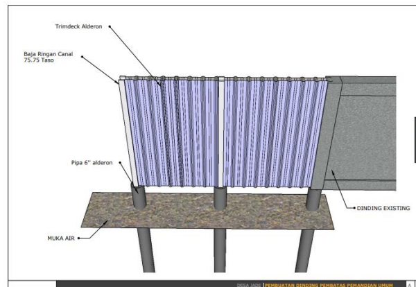
Gambar 4. Desain dinding tempat pemandian umum
