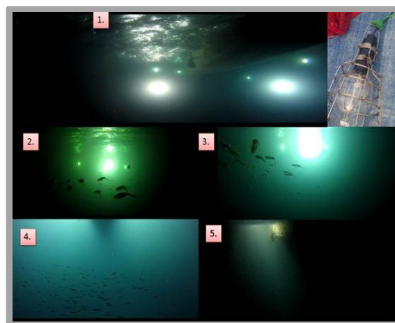
Gambar 3. Daya tembus cahaya pada saat penelitian.
