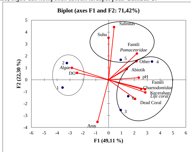
Gambar 3. Diagram hasil analisis komponen utama perairan Bedukang
