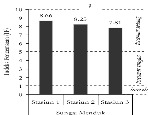
Gambar 3. Grafik (a) Indeks Pencemaran, (b) Indeks Habitat pada Stasiun Pengamatan
