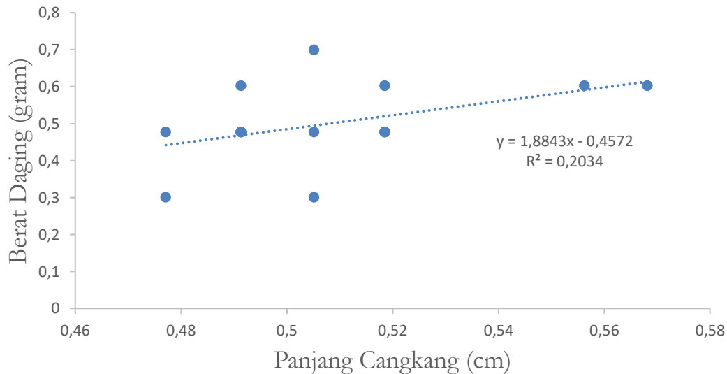
Gambar 3. Grafik Hubungan Panjang dan Berat Daging Kerang Darah
