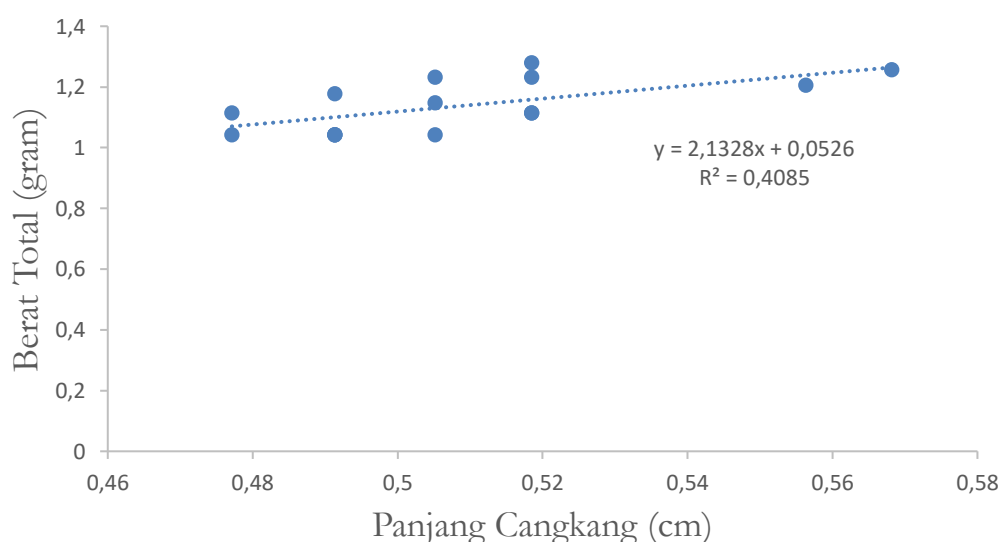
Gambar 2. Grafik Hubungan Panjang dan Berat Total Kerang Darah
