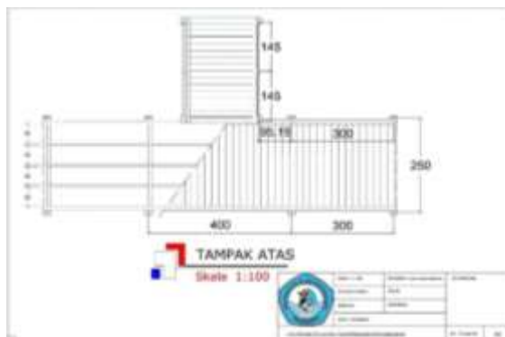
Gambar 6. Desain tampak atas dermaga kano (canoe docks).
