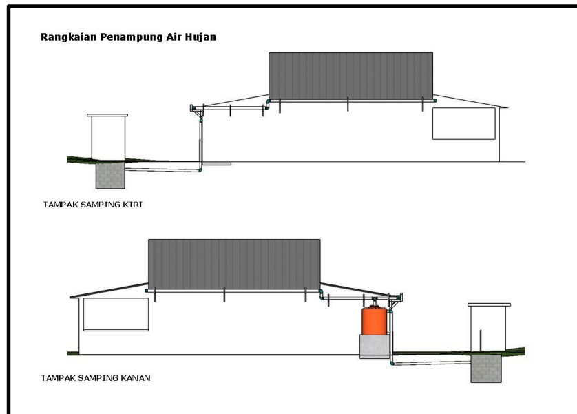
Gambar 4. Tampak Samping Letak Penampung Air Hujan (PAH)
