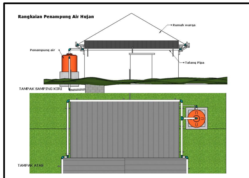
Gambar 5. Tampak Atas Instalasi PAH
