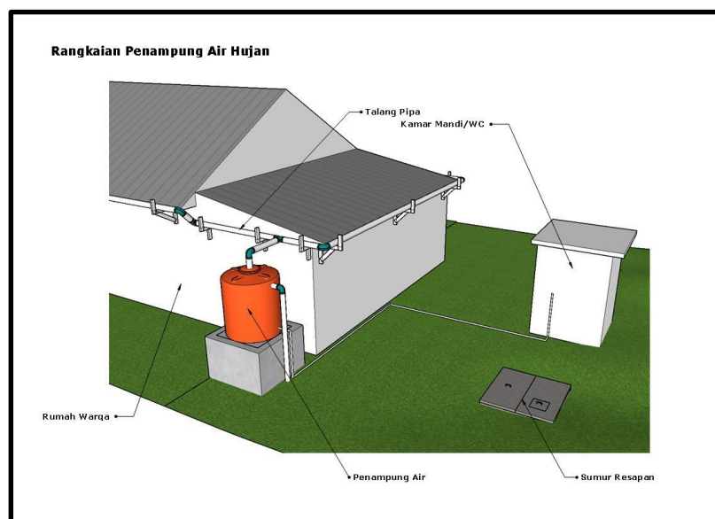
Gambar 6. Letak PAH dan Sumur Resapan Terhadap Septik Tank
