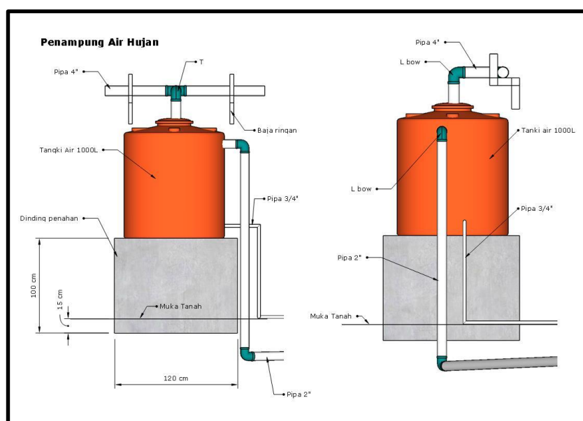
Gambar 3. Detail Penampung Air Hujan (PAH)
