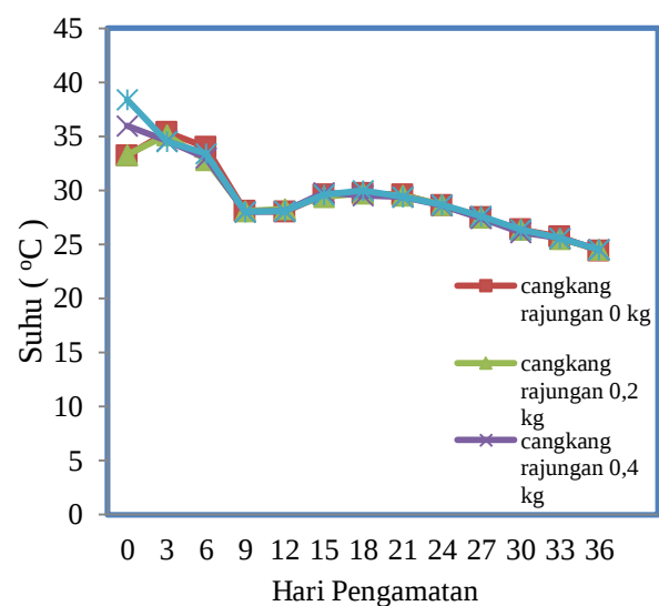
Gambar1. Grafik pengukuran Suhu kompos selama 36 hari.
