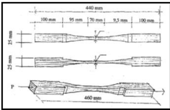
Gambar 6. Bentuk uji tarik material kayu
