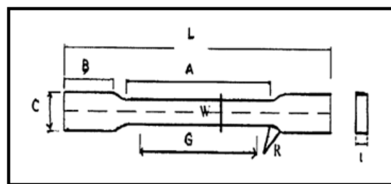
Gambar 1. Bentuk spesimen uji tarik material baja ringan
