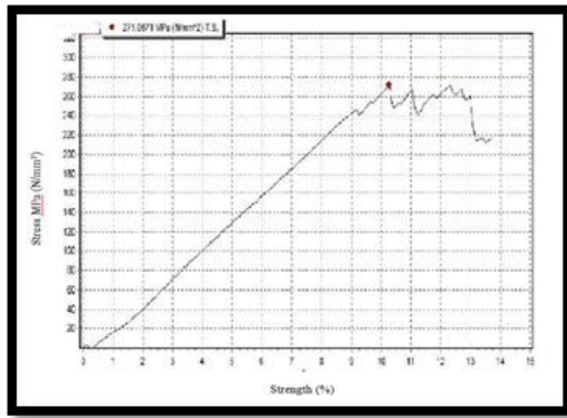
Gambar 9. Kurva tegangan dan regangan hasil pengujian sampel pertama Kayu Menggeris
