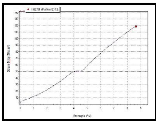
Gambar 10. kurva tegangan dan regangan hasil pengujian sampel pertama Kayu Nyato.
