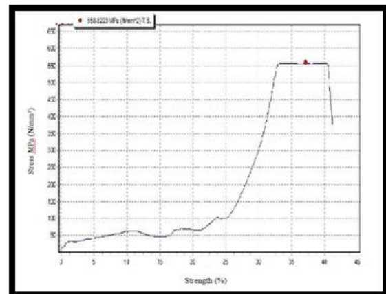
Gambar 4. Kurva tegangan dan regangan hasil pengujian sampel pertama C 7,5/0,75
