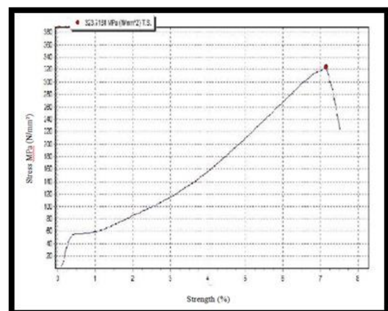
Gambar 5. Kurva tegangan dan regangan hasil pengujian sampel pertama profil U tebal 0,45.
