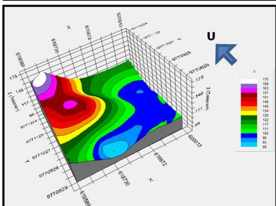
Gambar 6. Hasil analisis spasial data tahanan konus ( q_c ) menggunakan Ordinary Kriging (OK) 2D dan 3D.
