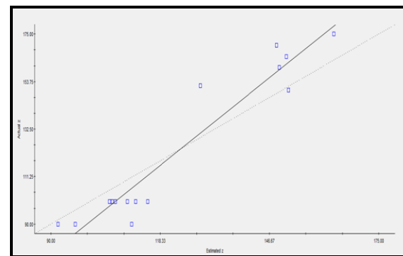
Gambar 7. Validasi silang data tahanan konus ( q_c )
