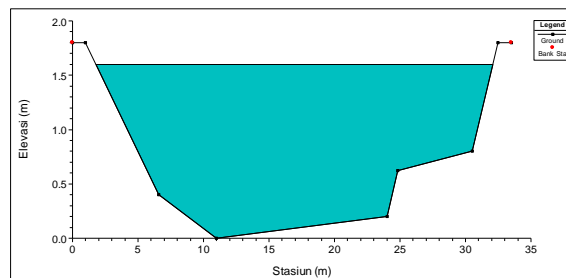
Gambar 5. Penampang melintang sungai bagian hilir
