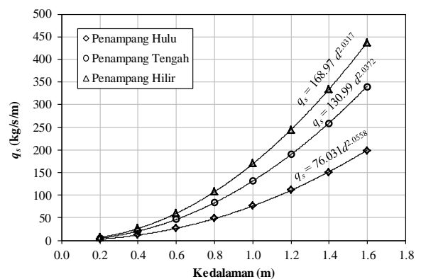
Gambar 11. Hubungan antara kedalaman ( d ) dan laju transpor material dasar per satuan lebar sungai ( q_s )
