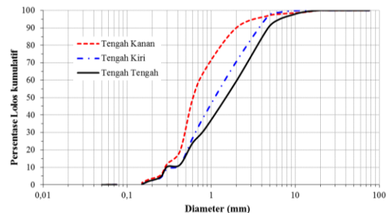
Gambar 8. Grafik gradasi butir sedimen bagian tengah
