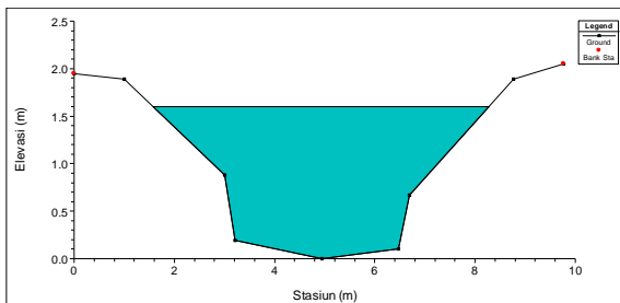
Gambar 3. Penampang melintang sungai bagian hulu
