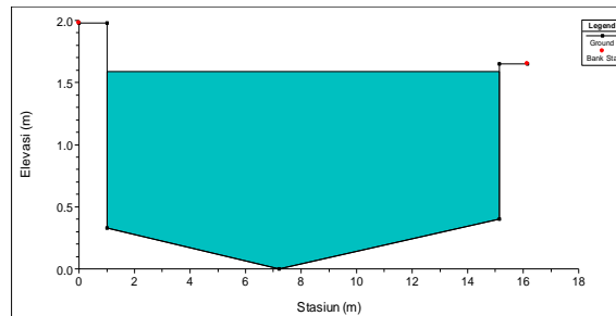
Gambar 4. Penampang melintang sungai bagian tengah
