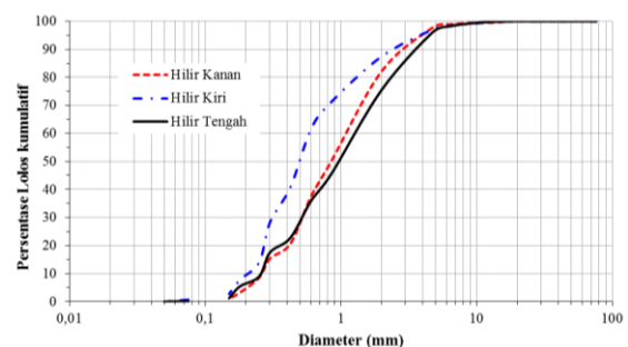
Gambar 9. Grafik gradasi butir sedimen bagian hilir
