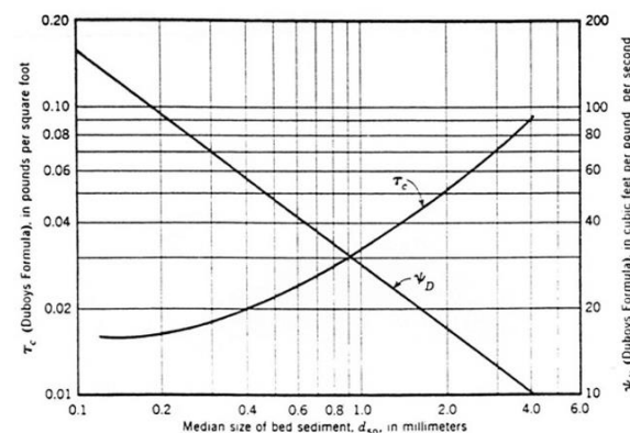
Gambar 1. Nilai \Psi_D dan \tau_c yang digunakan pada Persamaan Duboys
