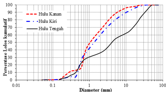
Gambar 7. Grafik gradasi butir sedimen bagian hulu
