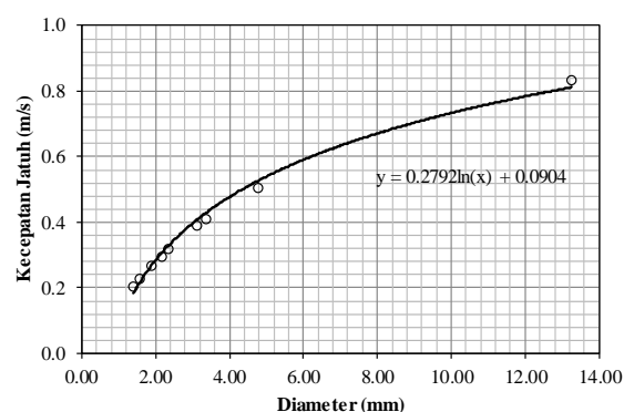
Gambar 10. Hubungan antara diameter rerata ( D_m ) dan kecepatan jatuh ( w ) partikel sedimen
