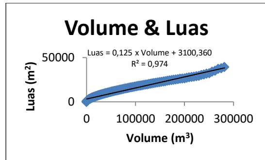
Gambar 7. Kurva hubungan antara volume tampungn terhadap luas permukaan tampungn
