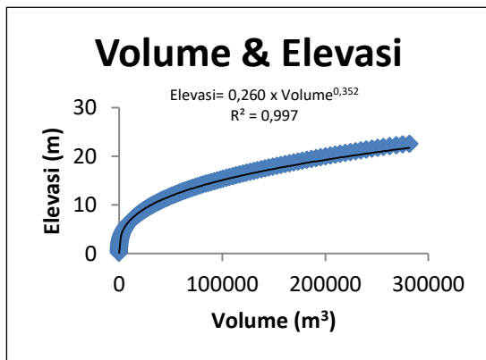
Gambar 5. Kurva hubungan antara volume tampungn terhadap elevasi
