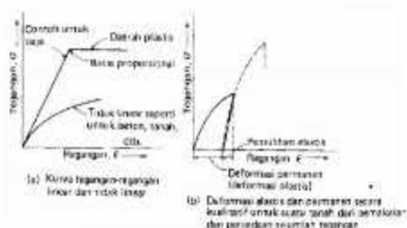
Gambar 1. Karakteristik Tegangan Regangan
