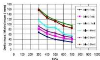
Gambar 4 Korelasi antara E/C_u dengan Deformasi Maksimum
