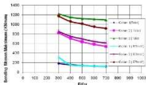
Gambar 6 Korelasi antara E/Cu dengan Bending Momen Maksimum
