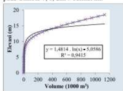
Gambar 7. Kurva hubungan volume terhadap elevasi kolom
