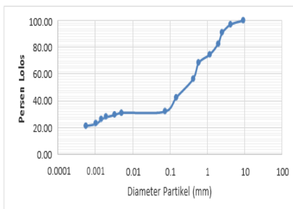
Gambar 2. Grafik Pengujian Hidrometer
