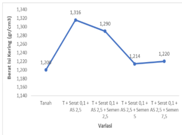
Gambar 4. Grafik Berat isi kering
