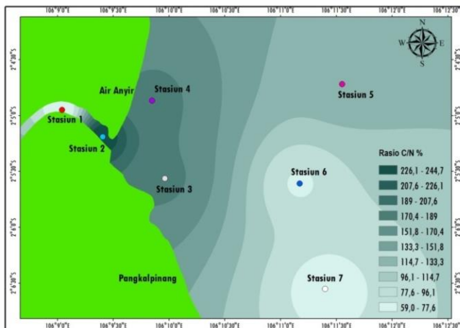
Gambar 4. Distribusi konsentrasi rasio C/N pada sedimen di Perairan Kawasan Pelabuhan Pangkal Balam
