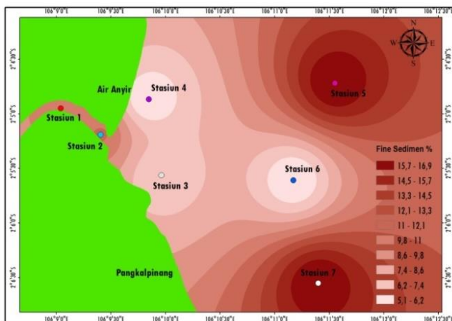
Gambar 5. Distribusi fine sediment di Perairan Kawasan Pelabuhan Pangkal Balam
