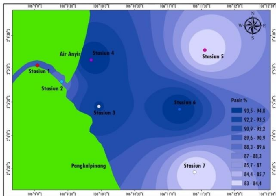
Gambar 6. Distribusi pasir di Perairan Kawasan Pelabuhan Pangkal Balam
