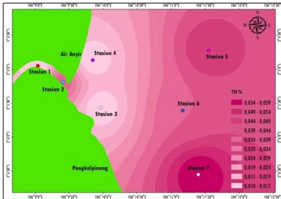
Gambar 3. Distribusi konsentrasi total nitrogen pada sedimen Perairan Baturusa
