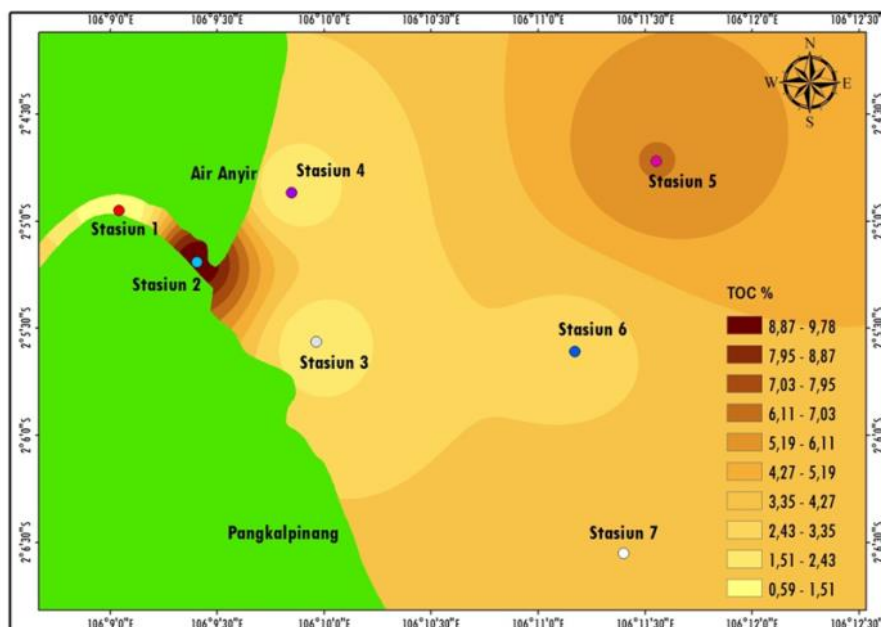
Gambar 2. Distribusi konsentrasi karbon organik total pada sedimen di Perairan Kawasan Pelabuhan Pangkal Balam
