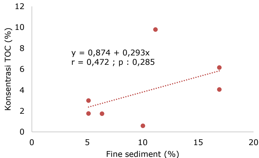
Gambar 7. Hubungan antara TOC (%) dengan fine sediment (%)
