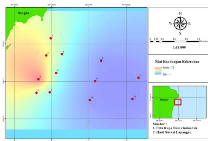
Gambar 2. Peta Sebaran Kekeruhan di Perairan Pantai Rebo, Kab. Bangka.
