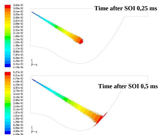
Gambar 4 Visualisasi penetrasi pada biodiesel MGB tekanan 175 bar
