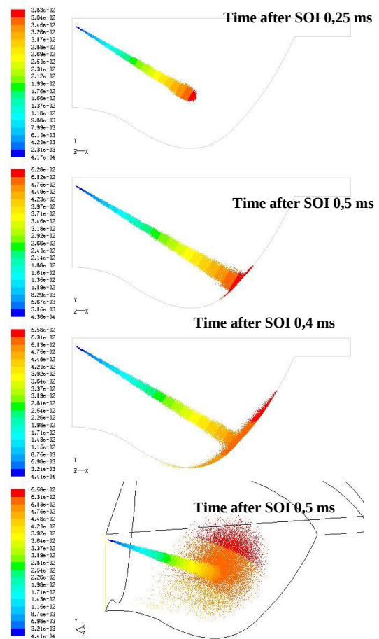
Gambar 4 Visualisasi penetrasi pada biodiesel MGB tekanan 175 bar
