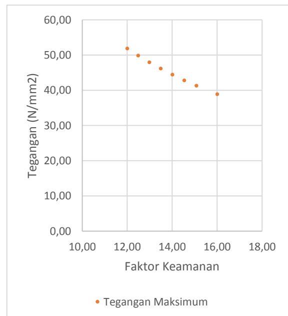
Gambar 8 Pengaruh faktor keamanan terhadap tegangan maksimum
