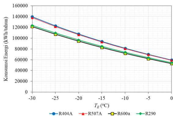
Gambar 12 Temperatur evaporasi vs konsumsi energi
