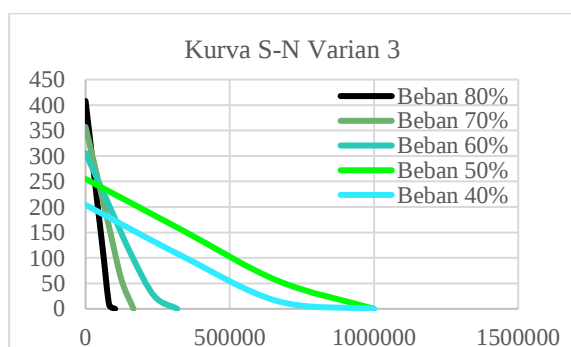
Gambar 7 Kurva S-N Varian 3
