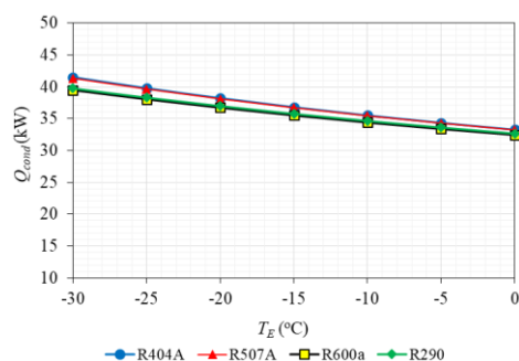
Gambar 9 Temperatur evaporasi vs pelepasan kalor di kondensor
