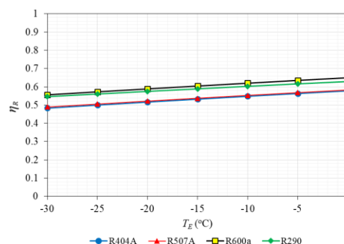
Gambar 11 Temperatur evaporasi vs efisiensi pendinginan
