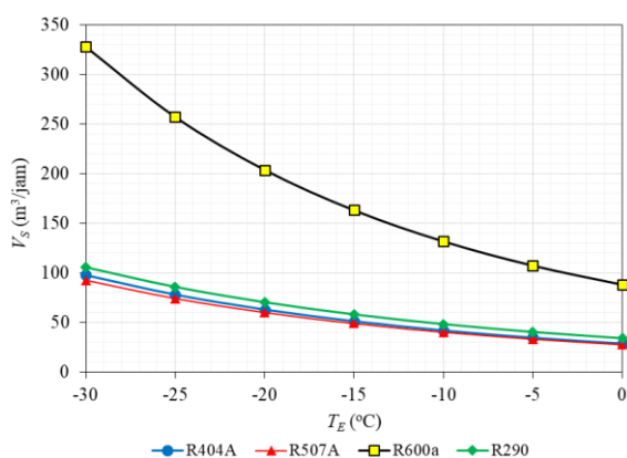
Gambar 13 Temperatur evaporasi vs volume hisap kompresor
