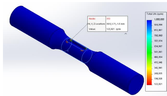
Gambar 3 Simulasi Uji Fatigue Rasio Alur Pasak 3:2
