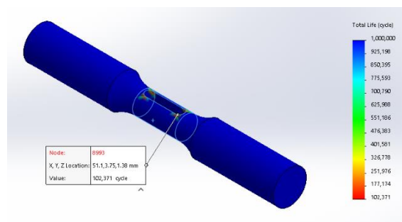
Gambar 4 Simulasi Uji Fatigue Rasio Alur Pasak 3:3
