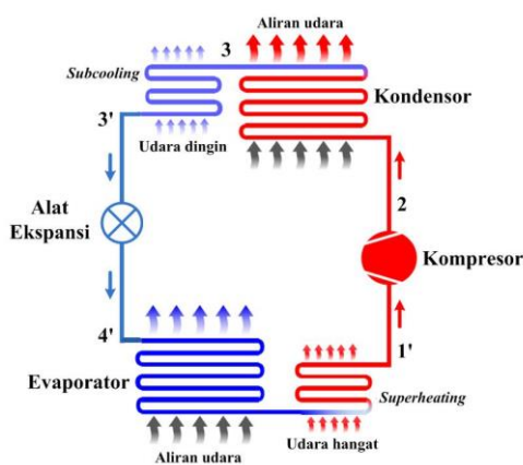
Gambar 2 Skematik refrigerator kompresi uap dengan subcooling dan superheating
