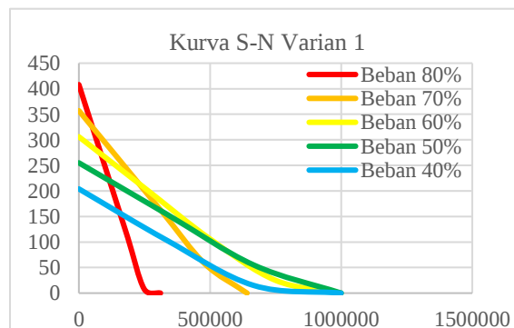
Gambar 5 Kurva S-N Varian 1
