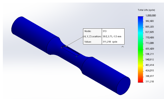
Gambar 2 Simulasi Uji Fatigue Rasio Alur Pasak 3:1
