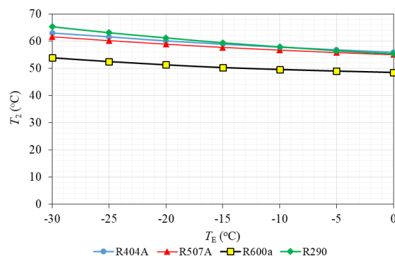
Gambar 7 Temperatur evaporasi vs temperatur gas refrigeran keluar kompresor
