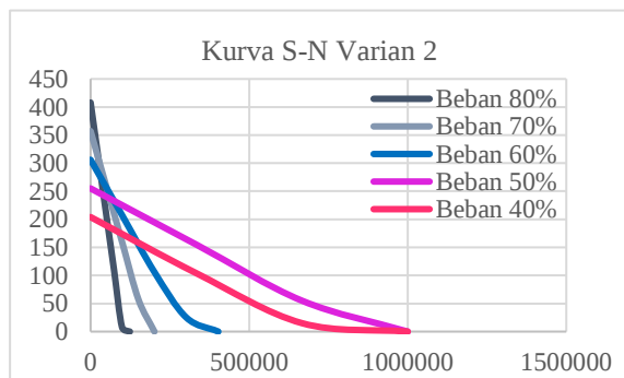
Gambar 6 Kurva S-N Varian 2
