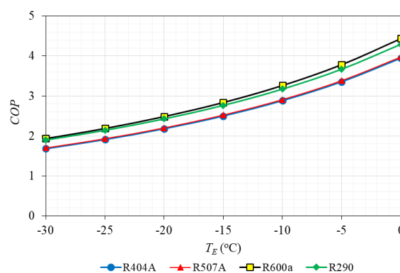
Gambar 10 Temperatur evaporasi vs koefisien kinerja
