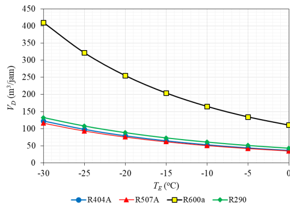
Gambar 14 Temperatur evaporasi vs volume buang kompresor
