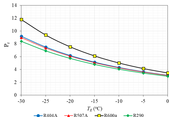
Gambar 6 Temperatur evaporasi vs rasio tekanan kompresor
