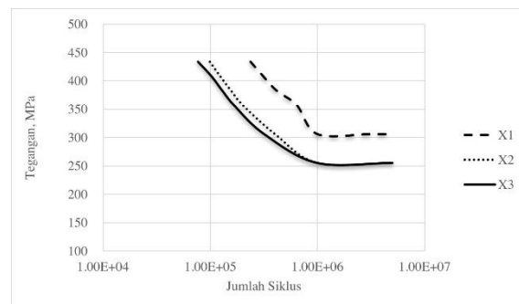
Gambar 8 Kurva S-N Beban 80%
