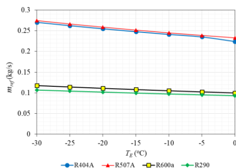
Gambar 5 Temperatur evaporasi vs laju aliran massa refrigeran
