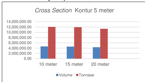
Gambar 6. Grafik hasil Metode Cross Section interval kontur 5 meter
