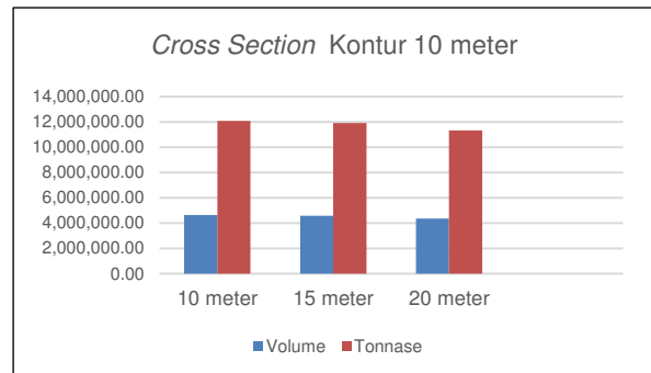
Gambar 7. Grafik hasil Metode Cross Section Interval Kontur 10 Meter
