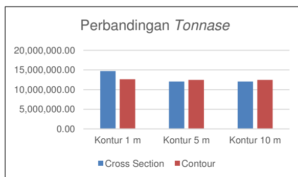
Gambar 10. Perbandingan tonnage Metode cross Section dan Metode Contour
