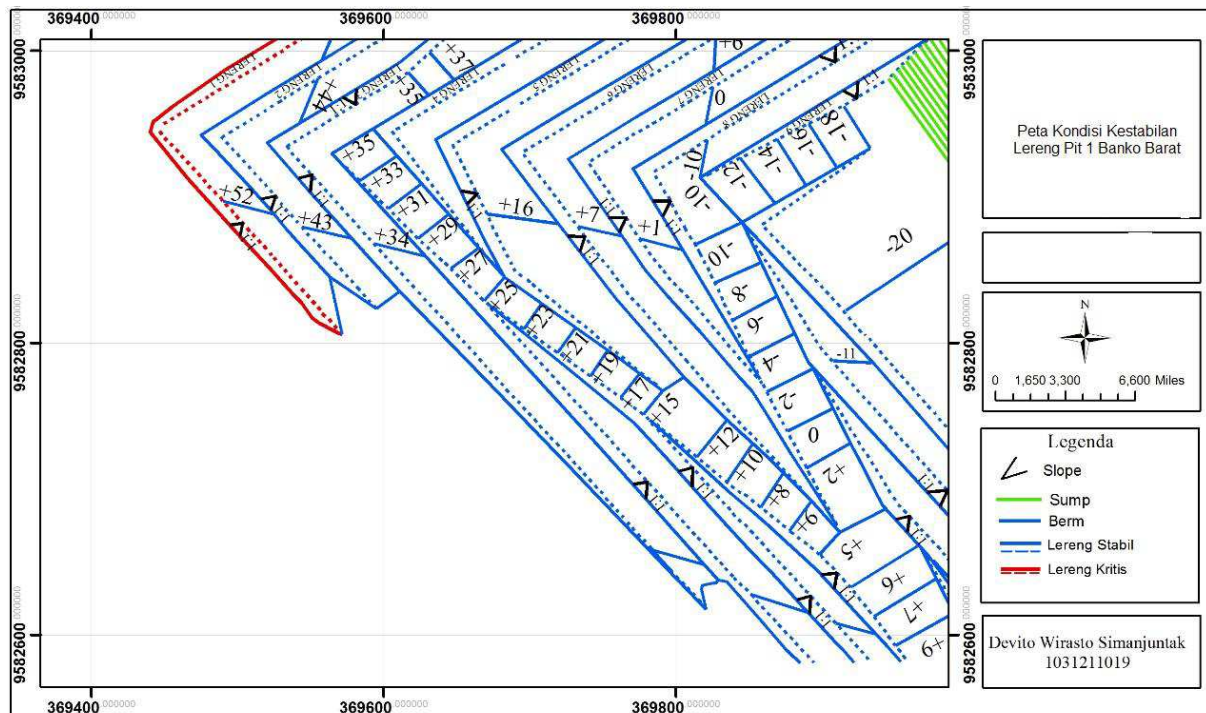
Gambar 3. Kondisi Kestabian Lereng Tunggal
