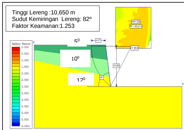
Gambar 3. Faktor keamanan
