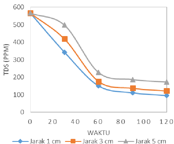
Gambar 3. Hubungan antara TDS dengan waktu elektrokoagulasi
