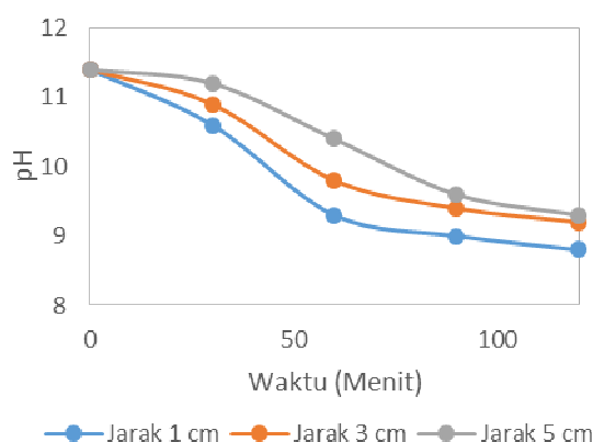
Gambar 2. Hubungan antara pH dengan waktu elektrokoagulasi
