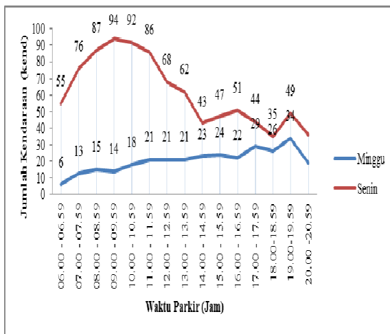
Gambar 3. Akumulasi Parkir Kendaraan Roda Empat
