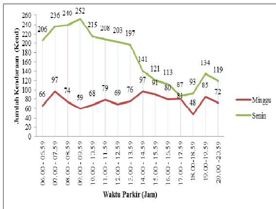
Gambar 2. Akumulasi Parkir Kendaraan Roda Dua
