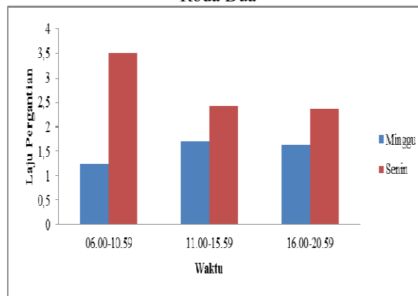
Gambar 11. Tingkat Pergantian Parkir Kendaraan Roda Empat
