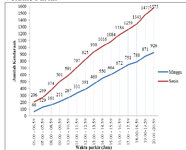
Gambar 4. Volume Parkir Kendaraan roda dua
