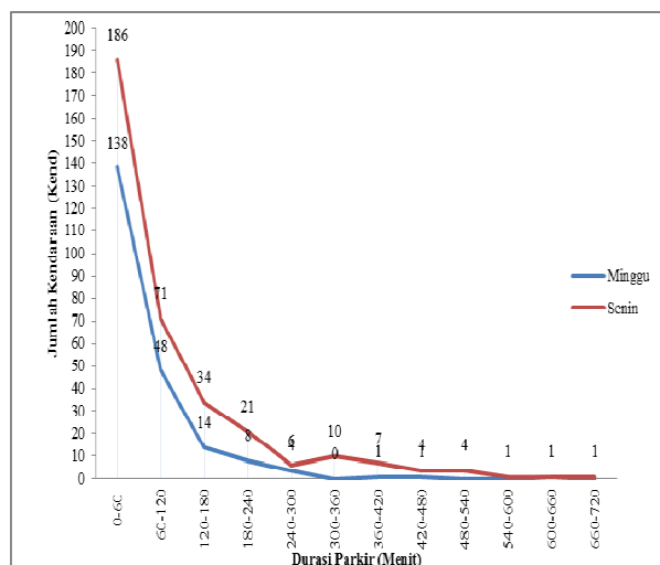
Gambar 7. Durasi Parkir kendaraan Roda Empat
