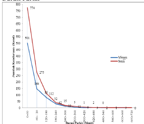
Gambar 6. Durasi Parkir Kendaraan Roda Dua
