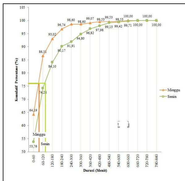
Gambar 8. Grafik Persentase Komulatif Kendaraan Roda Empat
