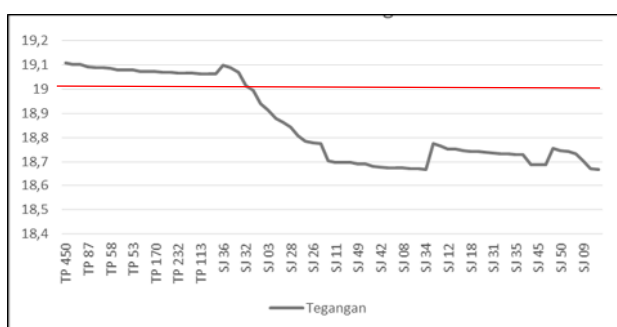
Gambar 1. Hubungan antara Tegangan Trafo di Penyulang metro
