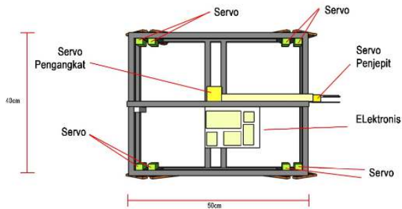
Gambar 3. Tampak Atas
