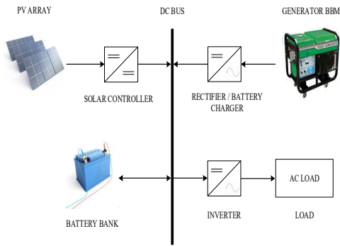
Gambar 1 Sistem Hibrid Seri
