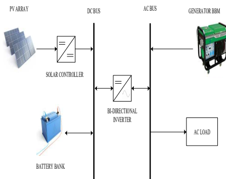
Gambar 3 Sistem Hibrid Paralel
