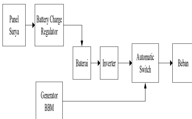
Gambar 4 Blok Diagram Perancangan
