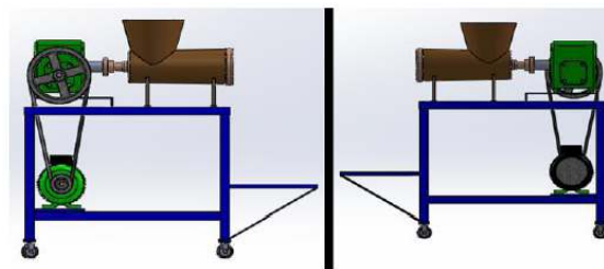
Gambar 3. Rancangan mesin penggiling daging ikan
