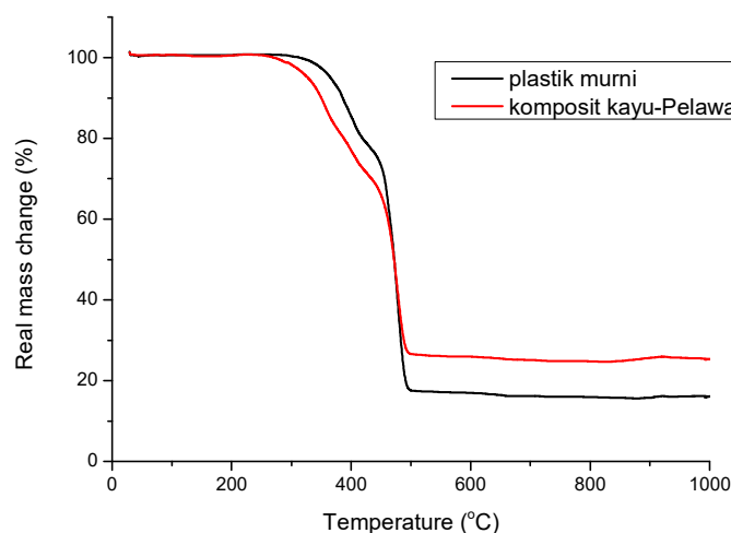
Gambar 3. Analisis Termal plastik murni dan komposit platik-serbuk kayu Pelawan
