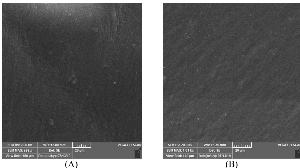
Gambar 2. Morfologi permukaan film (a) plastik yang telah dimurnikan, (b) material komposit sampah plastik dengan serbuk kayu Pelawan
