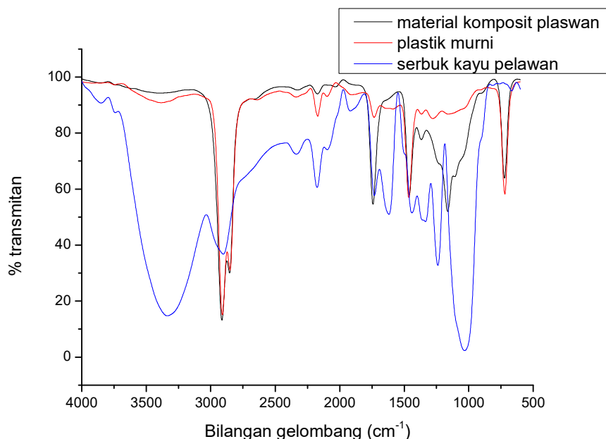
Gambar 1. Spektrum FTIR
