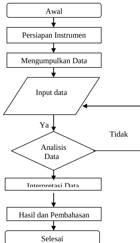
Gambar 1. Bagan alir tahapan penelitian
