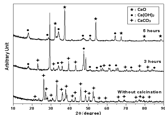
Gambar 2. Data Difraksi Cangkang Kerang
