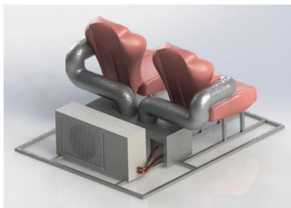
Gambar 4. Alat uji
