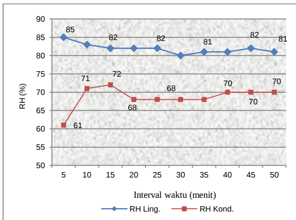
Gambar 6. Grafik kelembaban udara lingkungan dan udara yang dikondisikan sebagai fungsi interval waktu
