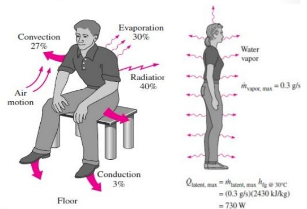
Gambar 3. Proses kehilangan kalor dari tubuh
