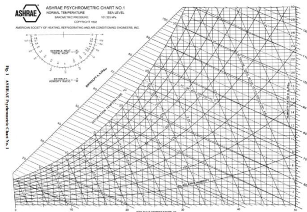
Gambar 1. Karta Psikrometrik
