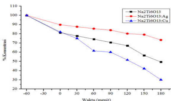
Gambar 6. Kurva perubahan konsentrasi MB terhadap lama waktu penyinaran.
