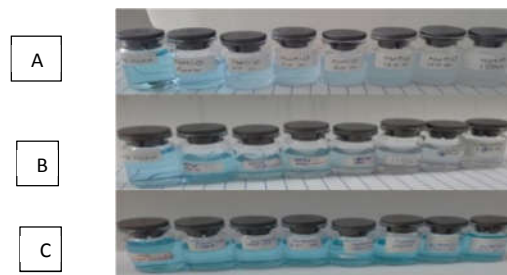
Gambar 4. Perubahan warna larutan MB setelah waktu iradiasi 3 jam menggunakan katalis (A) \text{Na}_2\text{Ti}_6\text{O}_{13} , (B) \text{Na}_2\text{Ti}_6\text{O}_{13}:\text{Cu} , (C) \text{Na}_2\text{Ti}_6\text{O}_{13}:\text{Ag} .
