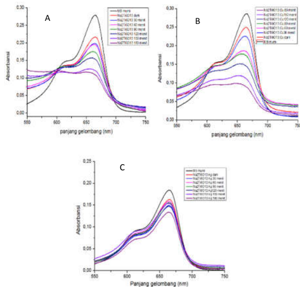
Gambar 5 Kurva absorbansi MB dibawah penyinaran sinar UV menggunakan katalis (A,) \text{Na}_2\text{Ti}_6\text{O}_{13} , (B) \text{Na}_2\text{Ti}_6\text{O}_{13}:\text{Cu} , (C) \text{Na}_2\text{Ti}_6\text{O}_{13}:\text{Ag} .
