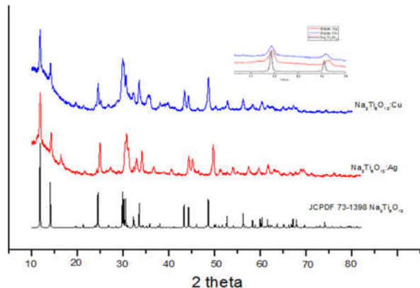
Gambar 3. Pola XRD \text{Na}_2\text{Ti}_6\text{O}_{13} terdopan ion \text{Cu}^{2+}/\text{Ag}^+
