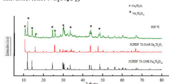
Gambar 1. Pola XRD \text{Na}_2\text{Ti}_6\text{O}_{13}
