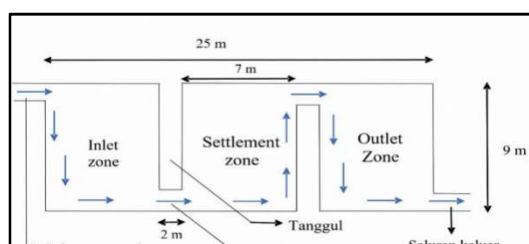
Gambar 4. Dimensi settling pond tampak atas
