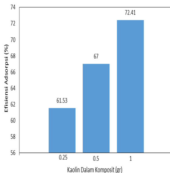
Gambar 1. Grafik Efisiensi Adsorpsi Ion Logam Cu 2+
