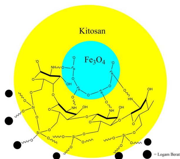
Gambar 3. Ilustrasi Reaksi Komposit \text{Fe}_3\text{O}_4 /Kitosan/Kaolin terhadap Logam Berat (Asriza dkk, 2019 dengan modifikasi).
