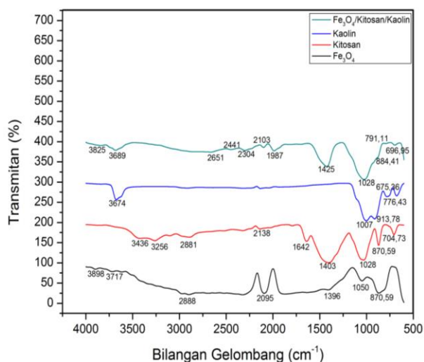
Gambar 2. Spektrum FTIR
