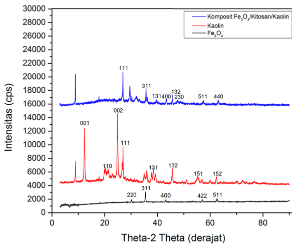
Gambar 4. Difraktogram XRD
