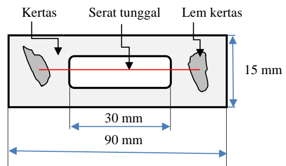
Gambar 4 Spesimen uji tarik serat alam
