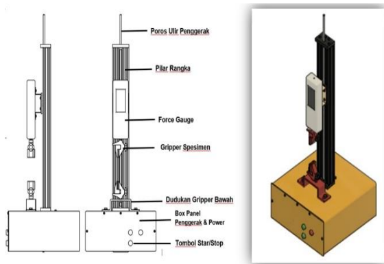
Gambar 1 Konsep rancangan alat uji tarik serat
